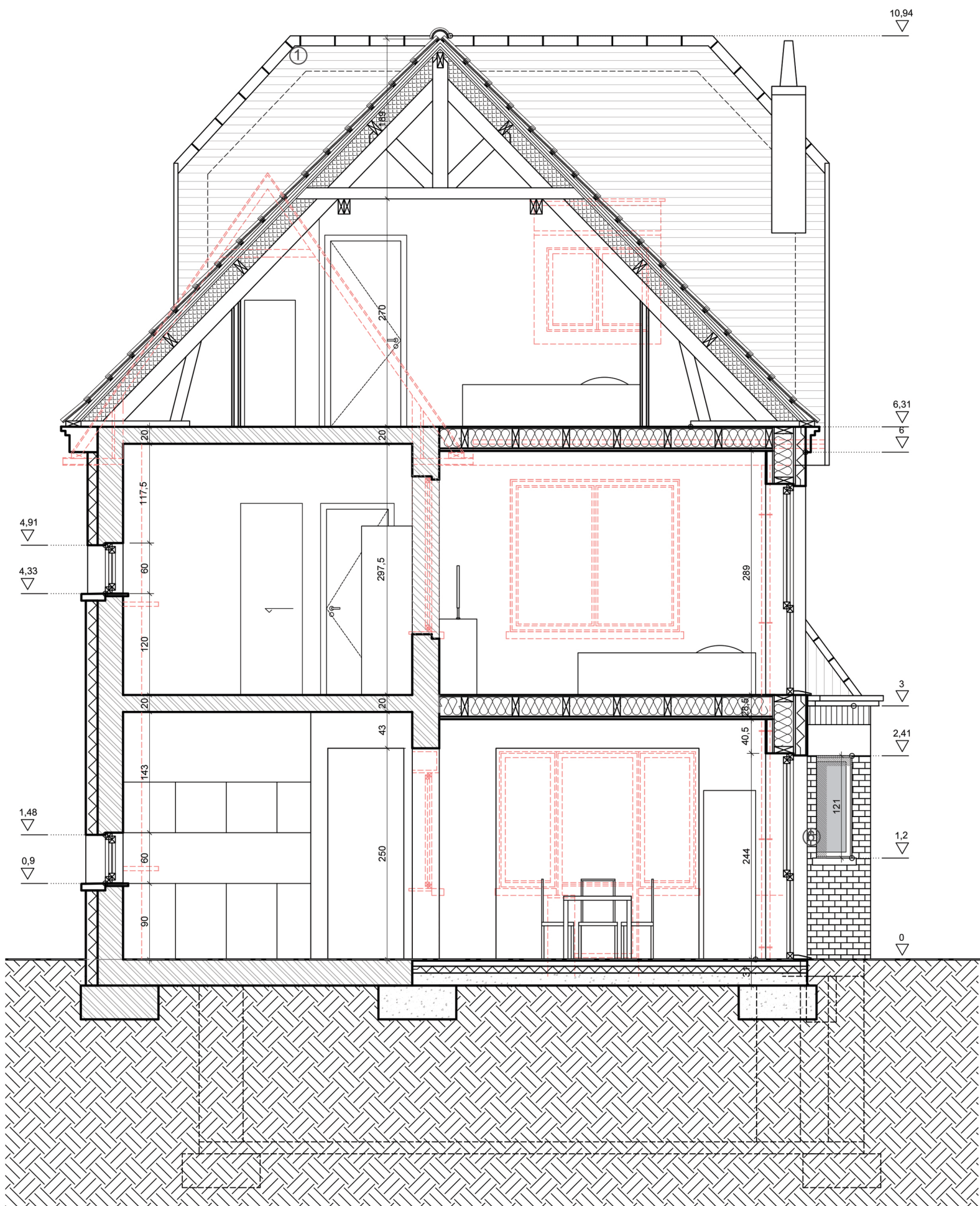
Coupe CC: 1/50e
